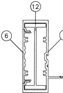
JAMB 'J2'
